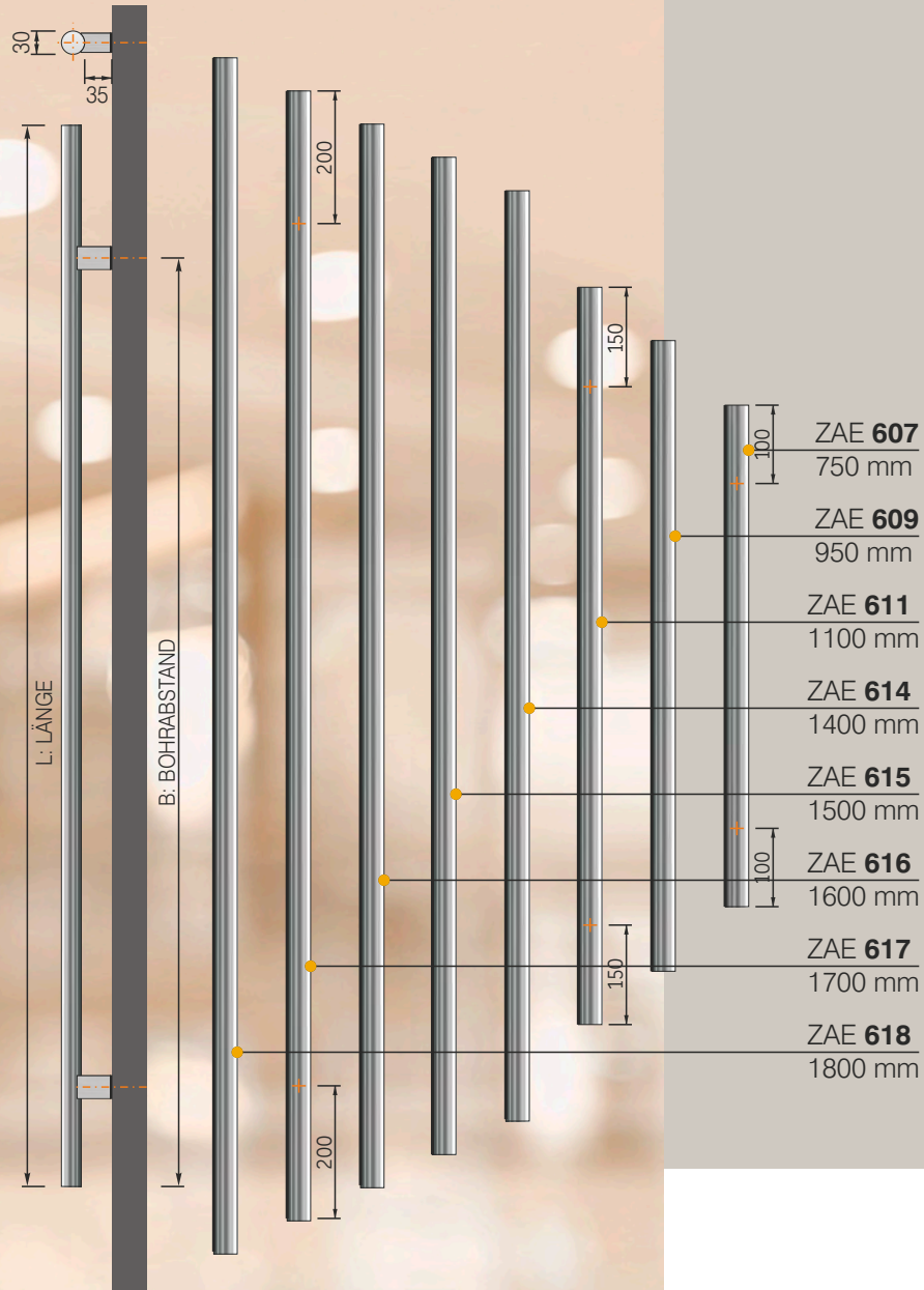
Stoßgriff Edelstahl matt
